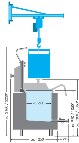
*Maße KA 240 für Gas und Öl
